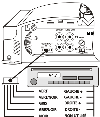
MGA265, MGA2100, MGA1190 ET MGA2150
