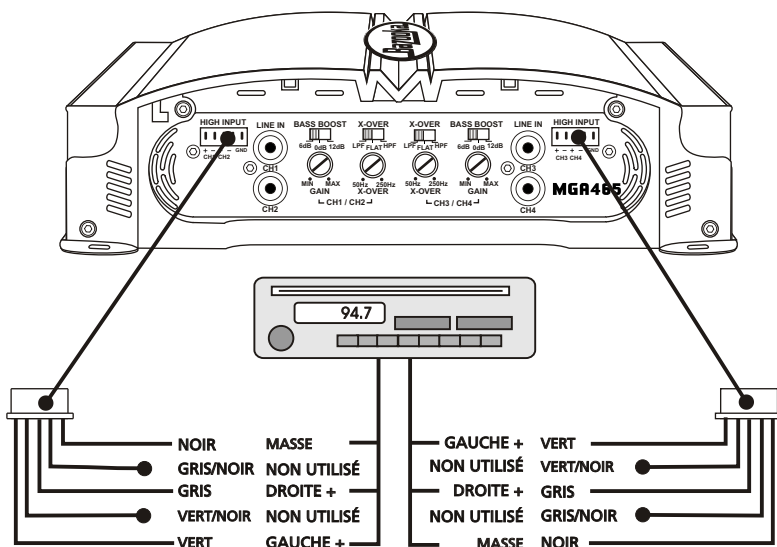
CONNEXIONS BR460 : RADIO EN CIRCUIT COMMUN ISOLÉ DE LA MASSE (TYPE LE PLUS COURANT)
