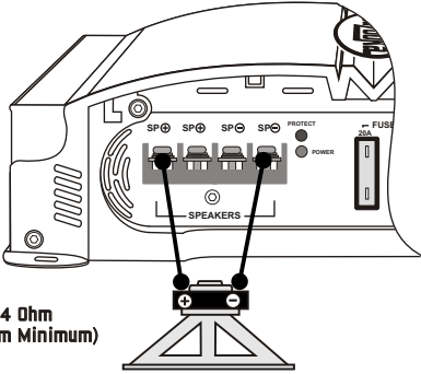
CONEXION DE BOCINAS: MGA1190, MGA1300, MGA1500 y MGA1800
