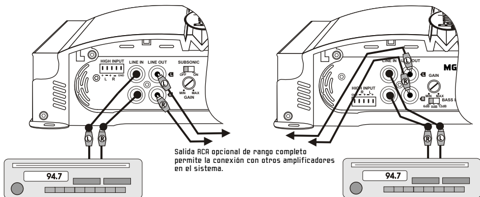
M6R265, M6R1190, M6R2100 y M6R2150 CONEXIONES DE SEÑAL
