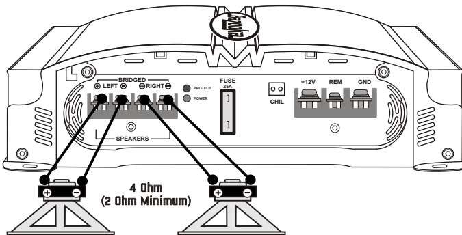
CONNEXIONS DES HAUT-PARLEURS MGA265, MGA2100 ET MGA2150
