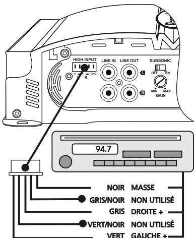
MGA1190, MGA1500 ET MGA1800
