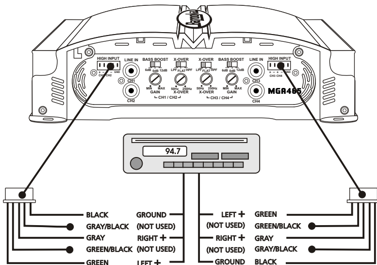
RADIO DE 4 CANALES CON TIERRA COMUN CON MGR465
