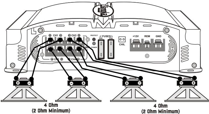
CONEXION DE BOCINAS: MGA465
