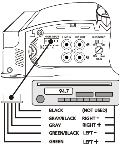
MGA1190, MGA1500 & MGA1800
