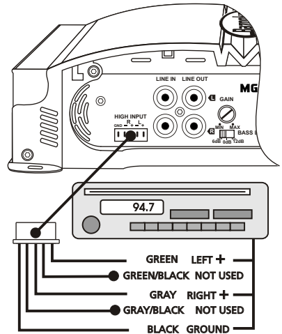
MGA265, MGA2100, MGA1190 & MGA2150
