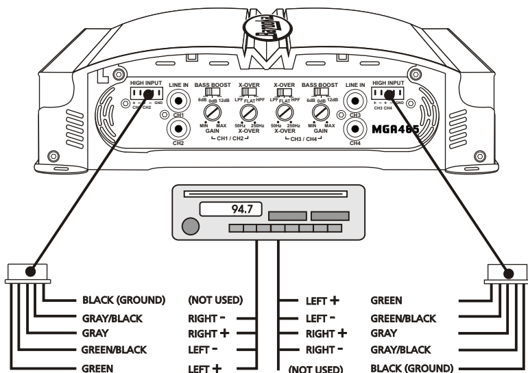
RADIO DE 4 CANALES CON TIERRA FLOTANTE CON MGR465
