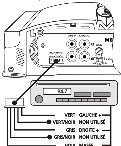
MGA265, MGA2100, MGA1190 ET MGA2150
