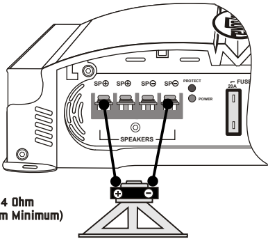
MGA1190, MGA1300, MGA1500 & MGA1800 SPEAKER CONNECTIONS
