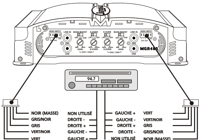
CONNEXIONS MGR465 : RADIO À MASSE COMMUNE
