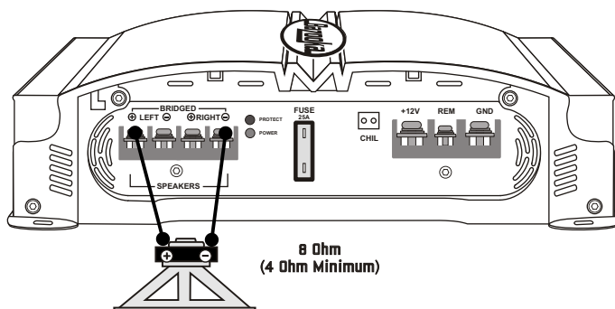
CONNEXIONS DES HAUT-PARLEURS EN DÉRIVATION MGA265, MGA2100 ET MGA2150
