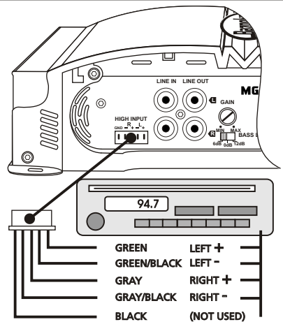
MGA265, MGA2100, MGA1190 & MGA2150
