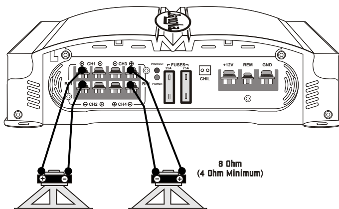
CONNEXIONS DES HAUT-PARLEURS EN DÉRIVATION MGA465
