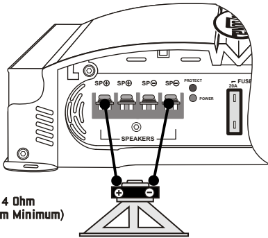
CONNEXIONS DES HAUT-PARLEURS MGA1190, MGA1300, MGA1500 ET MGA1800
