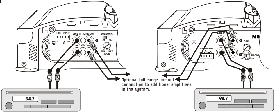
MGA1300, MGA1500, & MGA1800 SIGNAL CONNECTIONS
