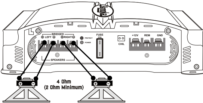
CONEXION DE BOCINAS: MGA265, MGA2100 y MGA2150
