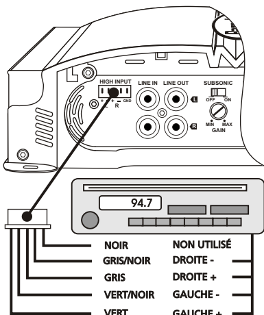
MGA1190, MGA1500 ET MGA1800
