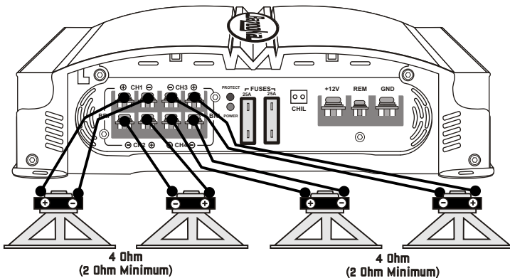
CONNEXIONS DES HAUT-PARLEURS MGA465
