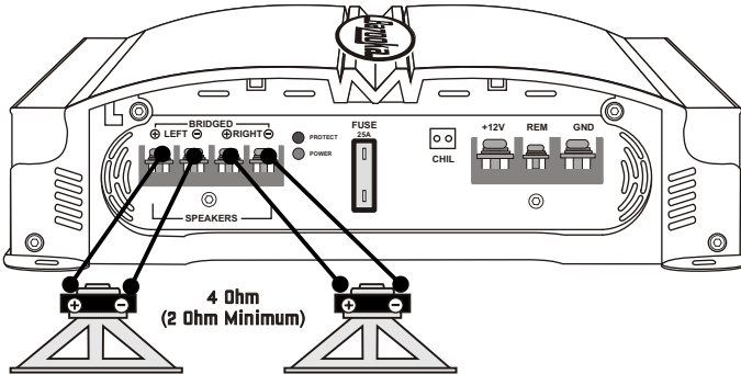
MGA265, MGA2100 & MGA2150 SPEAKER CONNECTIONS
